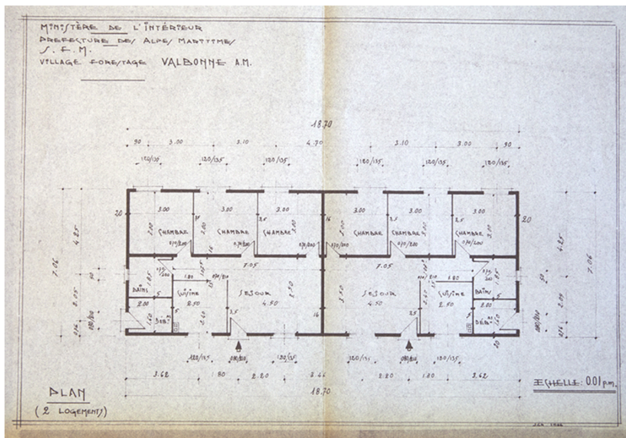
Plan (2 logements), 1966.
